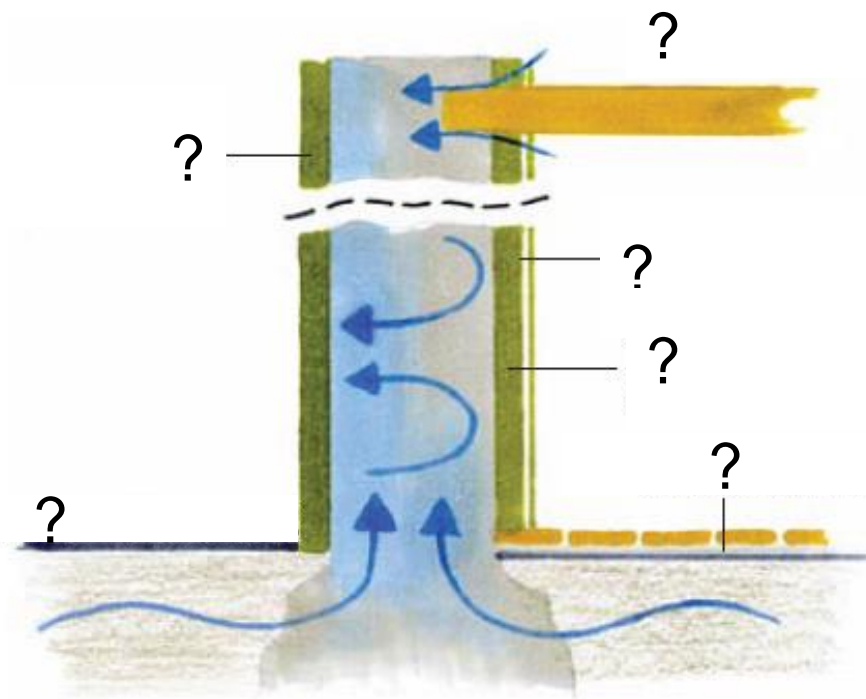
FONCTIONNEMENT HYGROMÉTRIQUE D'UN MUR TRADITIONNEL, ISOLÉ CONVENTIONNELLEMENT, EN HIVER: L'EAU S'ACCUMULE DANS LE MUR
