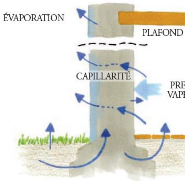
FONCTIONNEMENT HYGROMÉTRIQUE D'UN MUR TRADITIONNEL NON ISOLÉ
